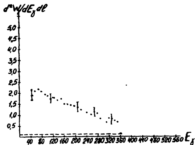
Рис.2 Спектр излучения электронов в режиме плоскостного каналирования в кристалле алмаза толщиной 1 мм
