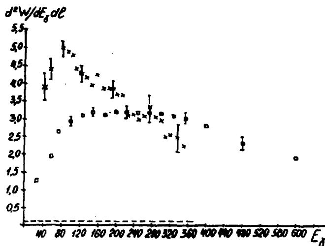
Рис.3 Спектры излучения электронов в режиме осевого каналирования в кристалле алмаза толщиной 1 мм
