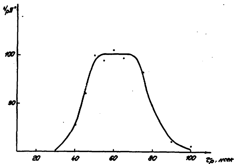
Рис.5 Кривая задержанных совпадений событий \rho\pi^0
