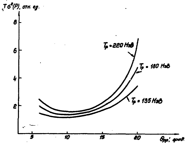
Рис.10 Зависимость T \cdot G^2(p) от угла наблюдения.
