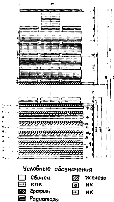
Рис.2 Схематический вид установки "Псион".
